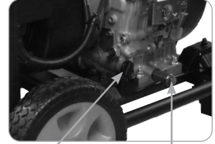
Ölmesstababdeckung Ablassabdeckung
