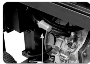
Kraftstofffilter
